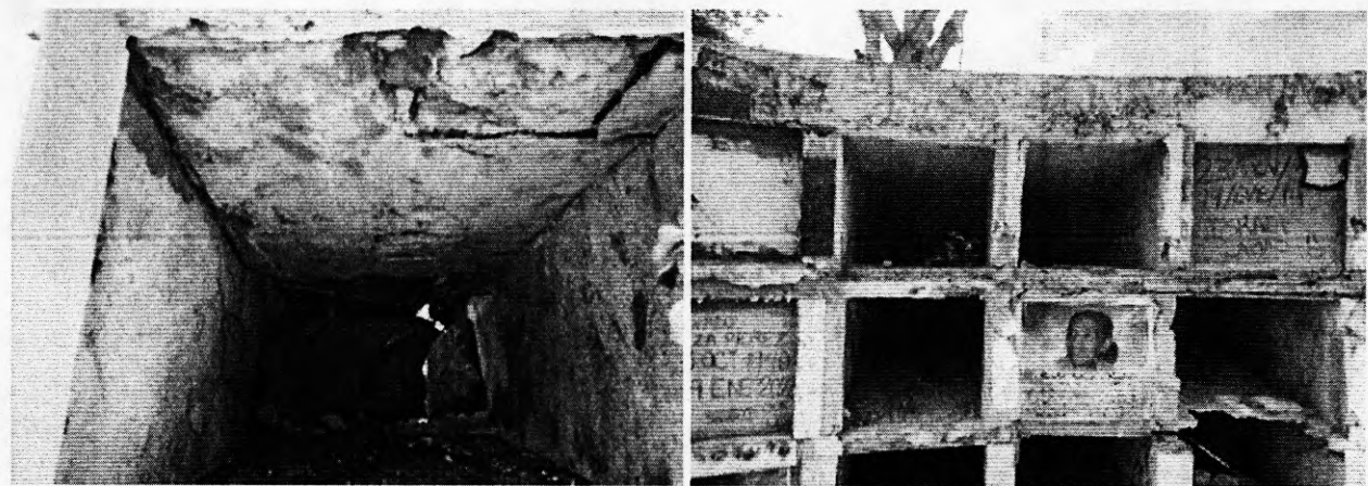
Figura 3. Estado de deterioro de modulo 7 de cementerio harmony hall para demolición
