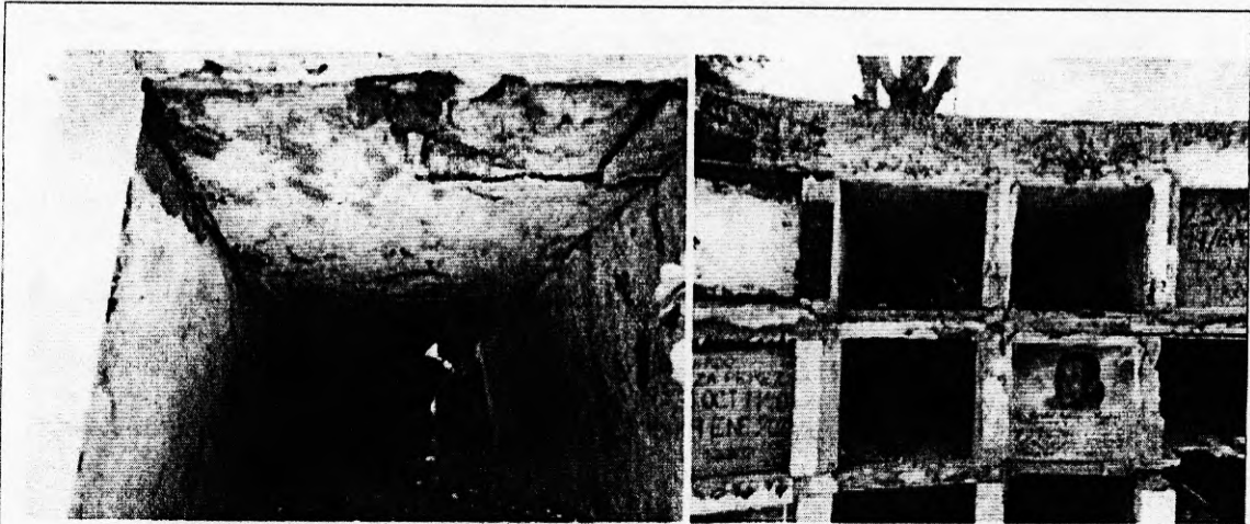
Figura 3. Estado de deterioro de modulo 7 de cementerio harmony hall para demolición
